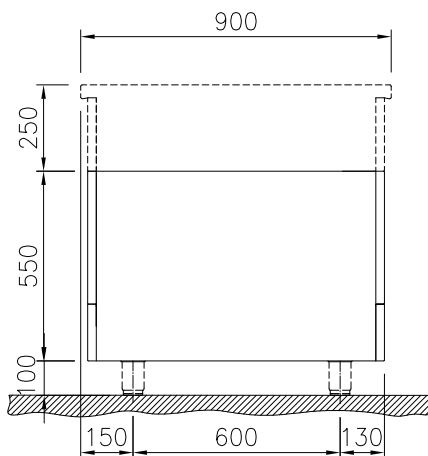
Boven aanzicht
